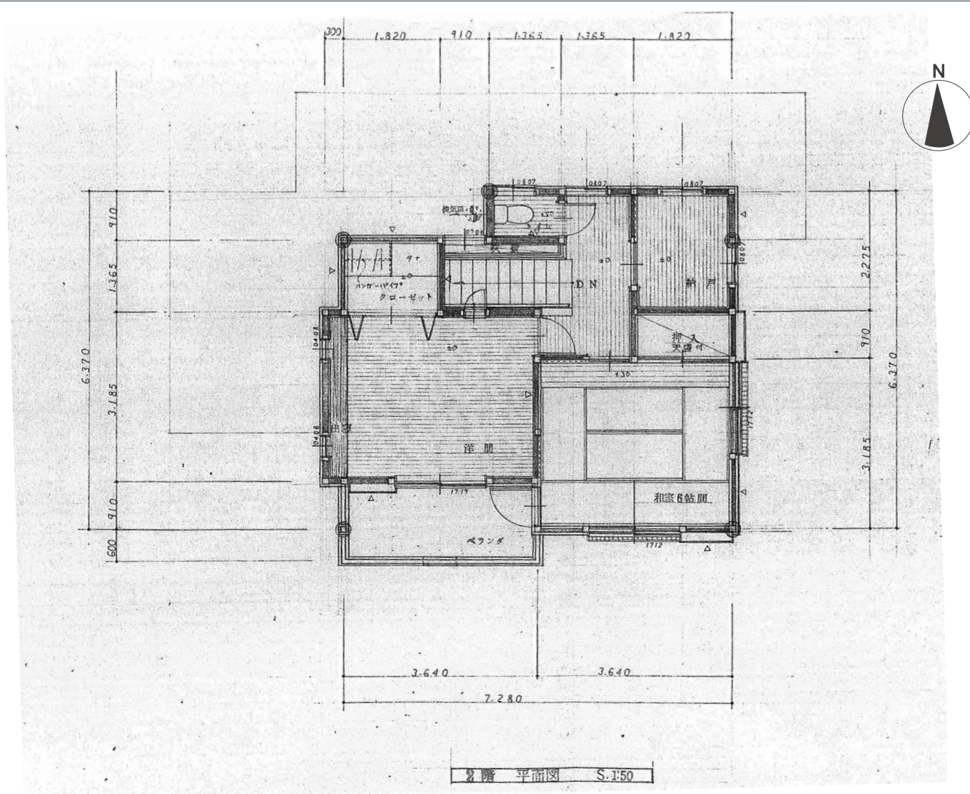
間取り図 2F
