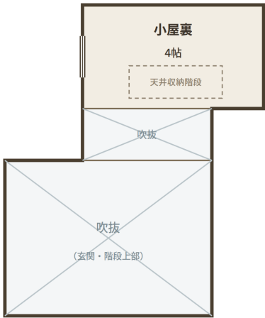
小屋裏平面図 小屋裏収納 4帖（2階上部）
